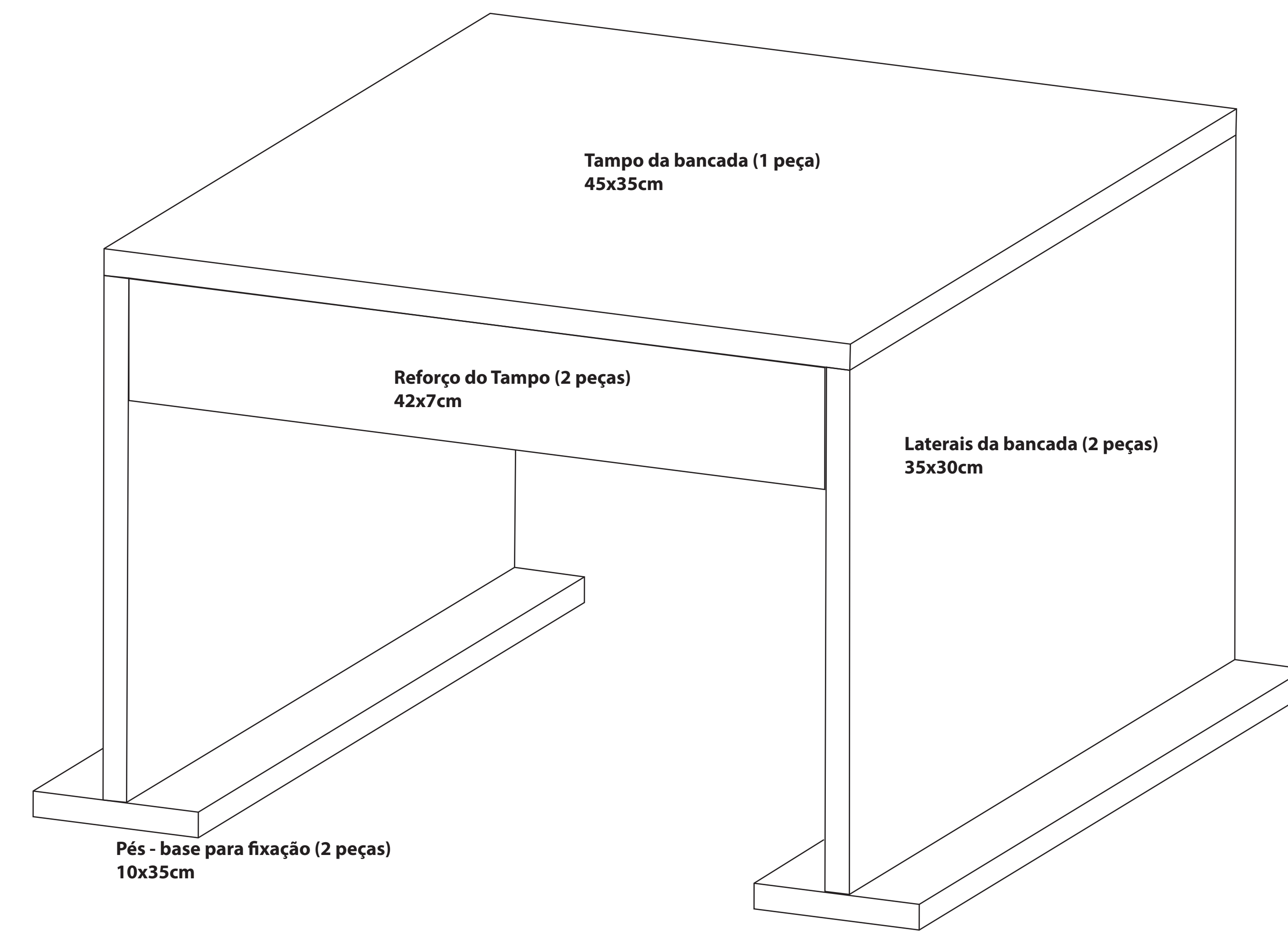
VISTA ISOMÉTRICA (Rascunho sem Escala - somente para visualização)
